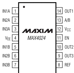
SO/TSSOP
