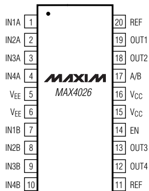
SO/TSSOP
