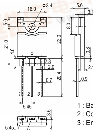
外形図 2174A
