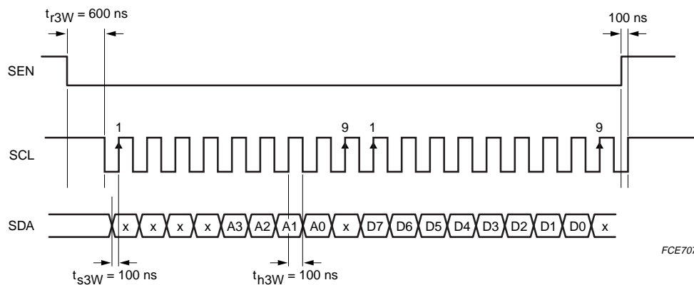
Fig 9. 3W-bus protocol.
