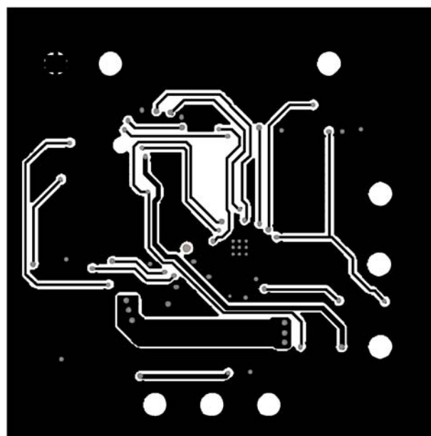
FIGURE 30. BOTTOM LAYER
