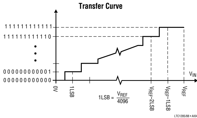
Output Code
