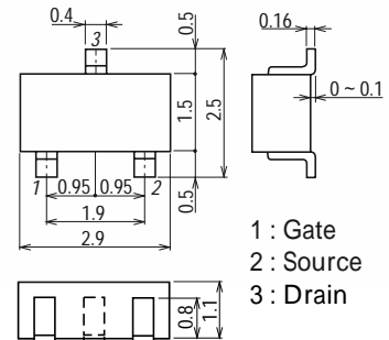
外形図 2091A
