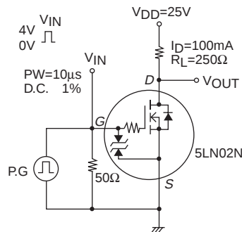
スイッチングタイム測定回路図
