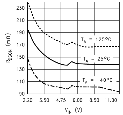
R_{DS(on)} vs. VIN ( I_{SW} = 1A )
