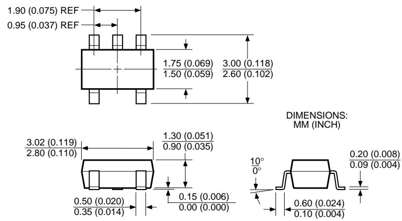
SOT-23-5 (M5)
