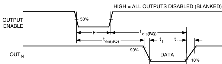
Dwg. WP-030-1
