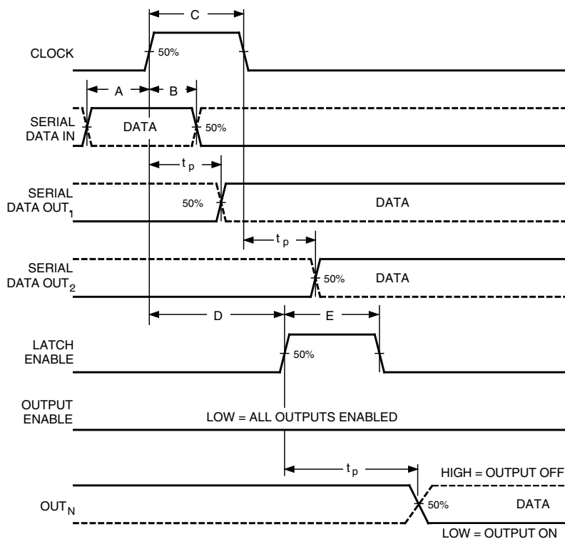
Dwg. WP-029-3
