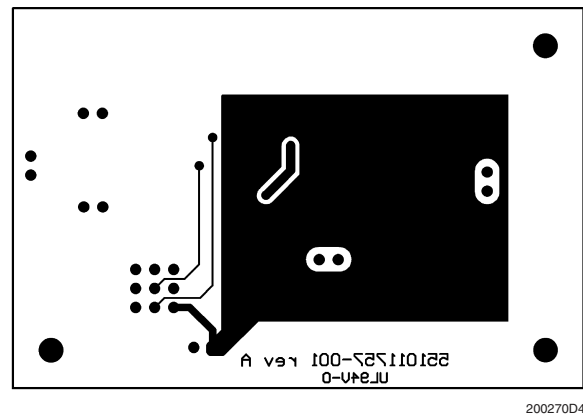
Bottom Layer
