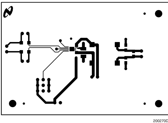
Top Layer
