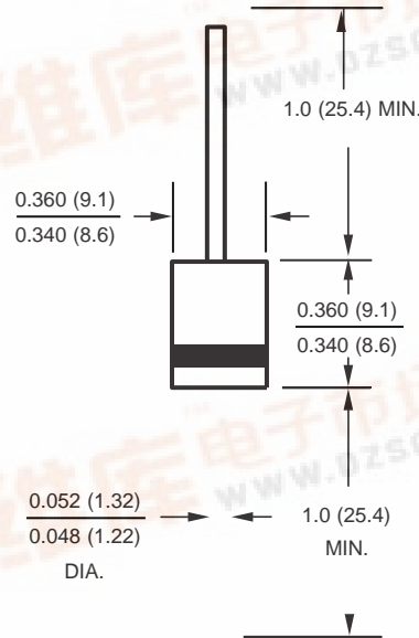
P600
