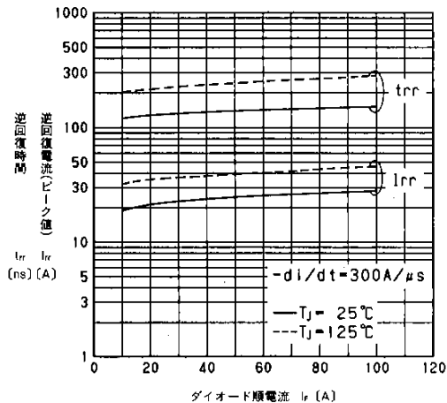
T_{rr} , I_{rr} - I_c 特性 T_{rr} , I_{rr} - I_c
