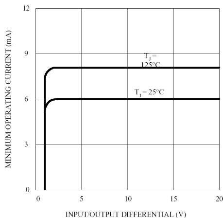
最小工作电流 (可调整稳压器)
