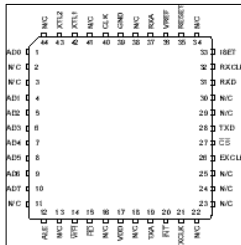
44-Lead TQFP 73K324L-IGT
