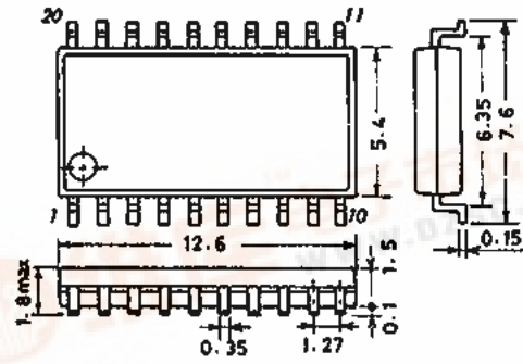
外形図 3036B-IC (LC7881M) (unit: mm)
