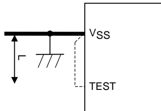
図19.TEST端子配線例
