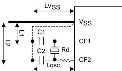
図16. 発振回路例1(セラミック発振使用時)
