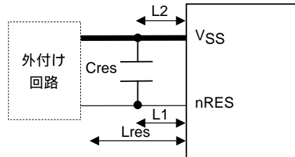
図18.nRES端子配線例
