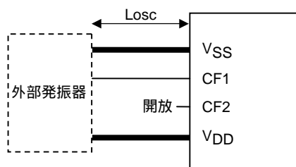
図17. 発振回路例2(外部発振器使用時)
