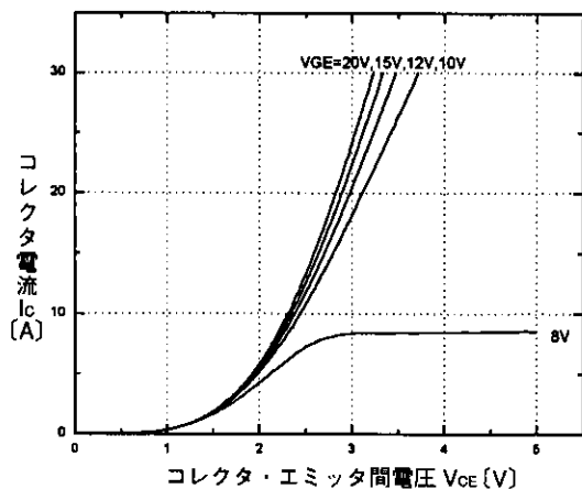
コレクタ電流—コレクタ・エミッタ間電圧特性 ( T_j = 25^\circ\text{C} ) <ブレーキ部> Collector current vs. Collector-Emitter voltage <BRAKE>
