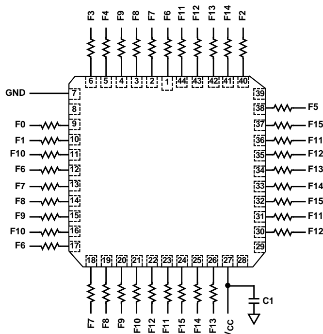
MR82C55A CLCC
