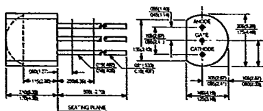
JEDEC TO-92
