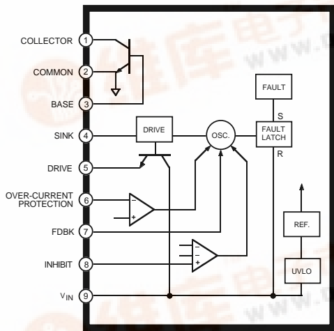
Dwg. PK-001
