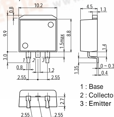
外形図 2069C
