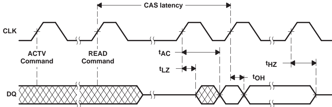
Figure 10. Output Parameters
