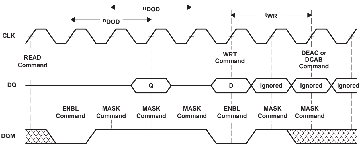
Figure 16. DQ Masking
