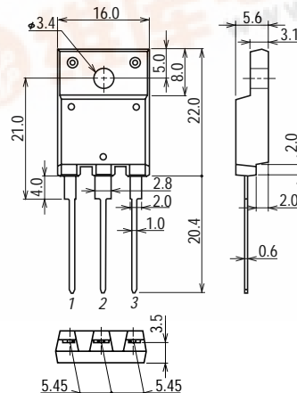
外形図 2039D
