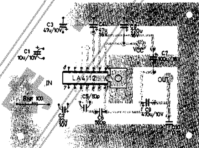
プリントパターン例(銅箔面)60×80mm 2
