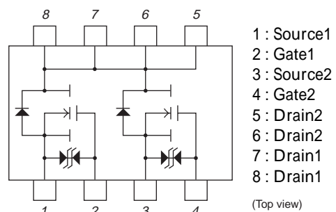
電気的接続図
