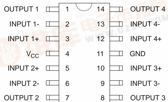
SOIC-14/DIP-14
