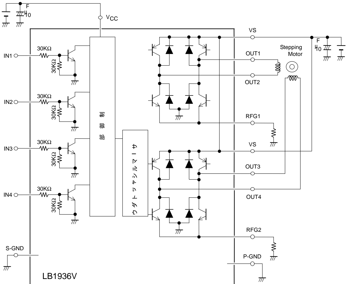
ブロック図
