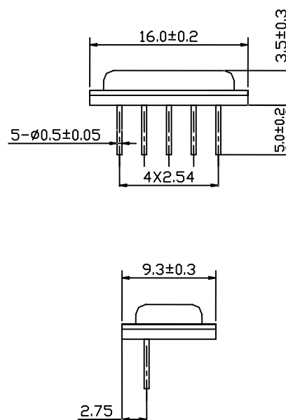
M (SF-915)
