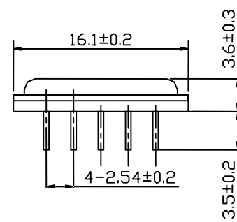
C (S-6BA)
