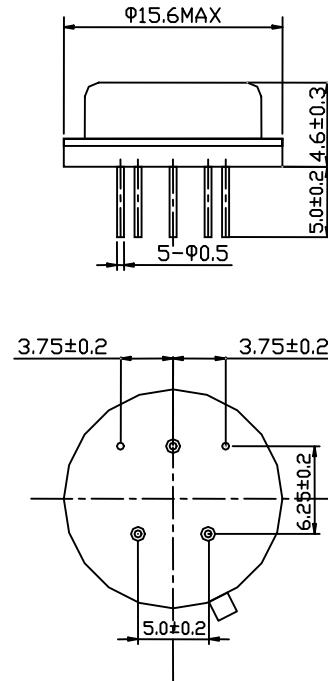
M (SF-915)
