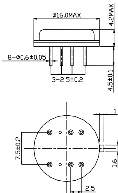
T (T-4)
