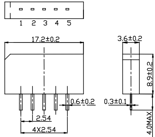
N (SIP5K)
