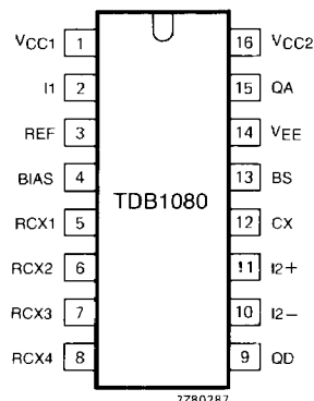
Fig. 2 Pinning diagram.
