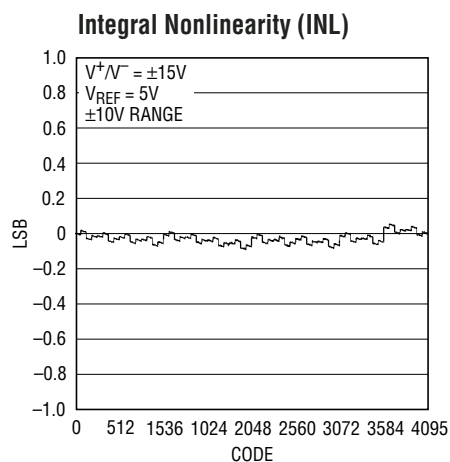
LTC2704-16/LTC2704-14/LTC2704-12
