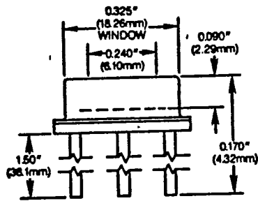
TO-5
