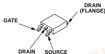
JEDEC TO-252AA
