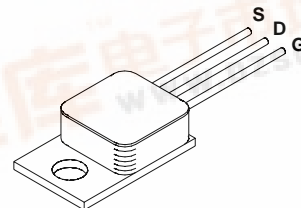
TO-257AA
