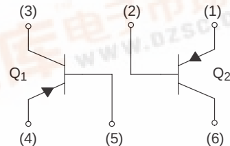
MBT3906DW1T1
