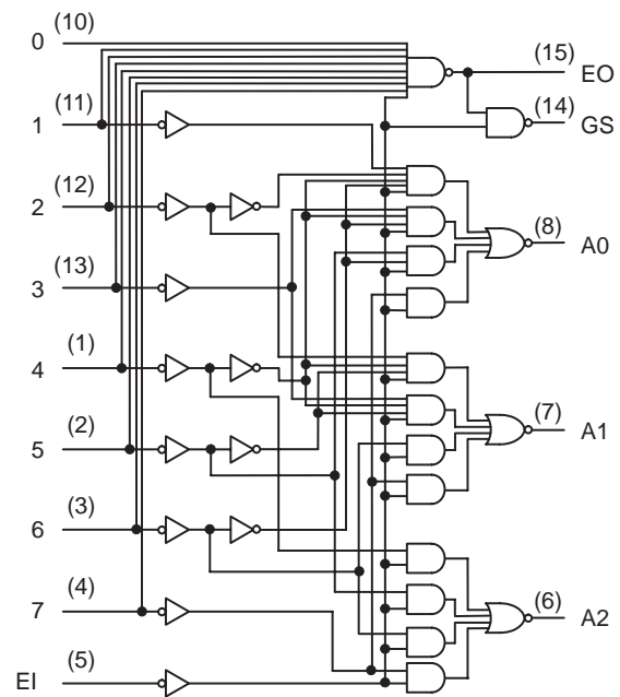
SN74LS148
