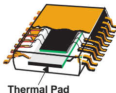
Thermal Pad
