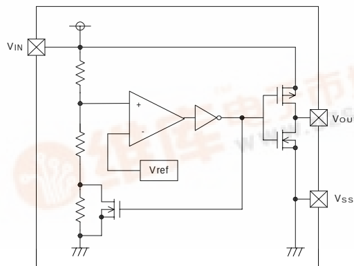
(1) CMOS Output
