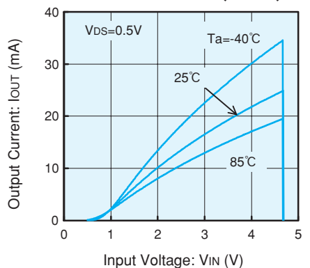
XC61CC4502 (4.5V)
