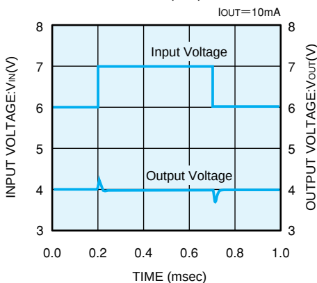
XC62HR4002 (4V)
