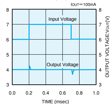
XC62HR4002 (4V)
