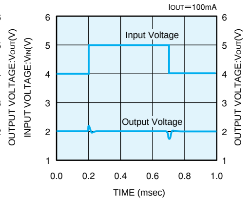
XC62HR2002 (2V)
