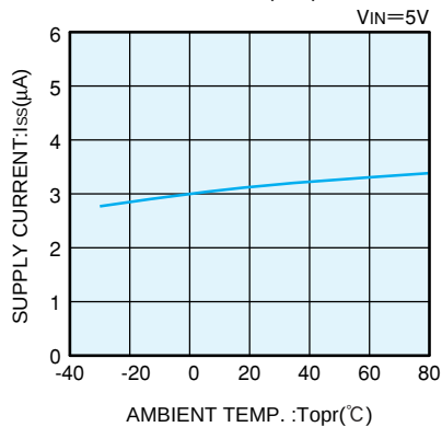
XC62HR4002 (4V)
