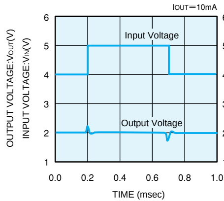
XC62HR2002 (2V)
