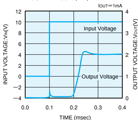
XC62HR2002 (2V)
