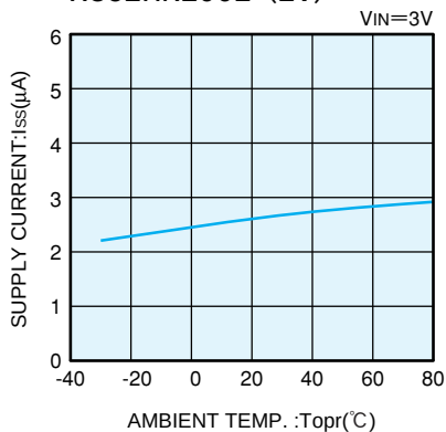
XC62HR2002 (2V)
