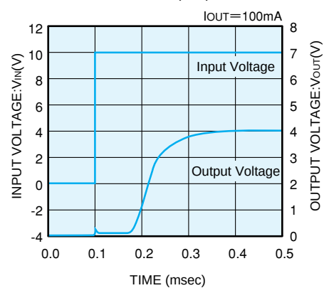
XC62HR4002 (4V)
