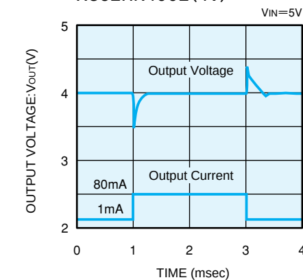
XC62HR4002 (4V)
