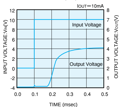
XC62HR4002 (4V)
