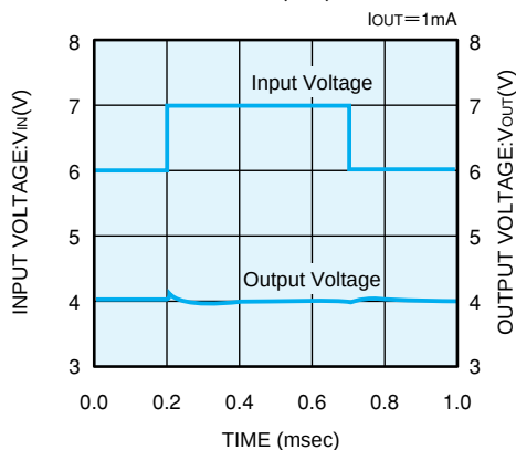
XC62HR4002 (4V)
