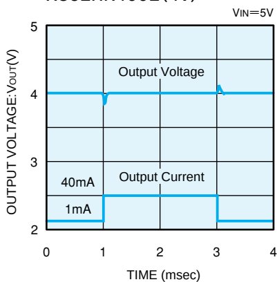
XC62HR4002 (4V)
