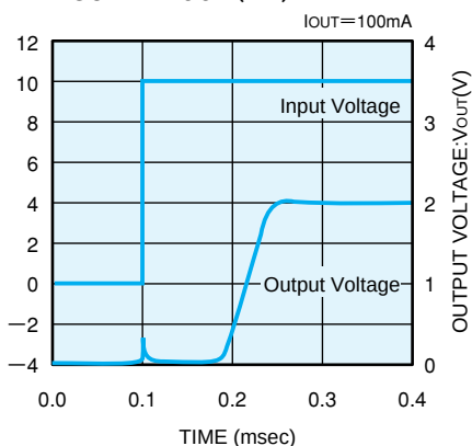
XC62HR2002 (2V)
