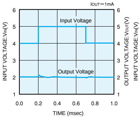
XC62HR2002 (2V)
