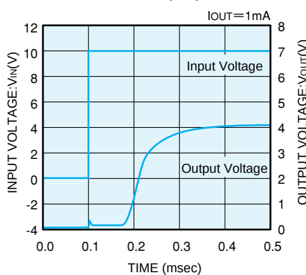
XC62HR4002 (4V)
