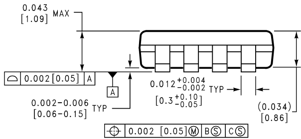
Mini SO-8 Package NS Package Number MUA08A
