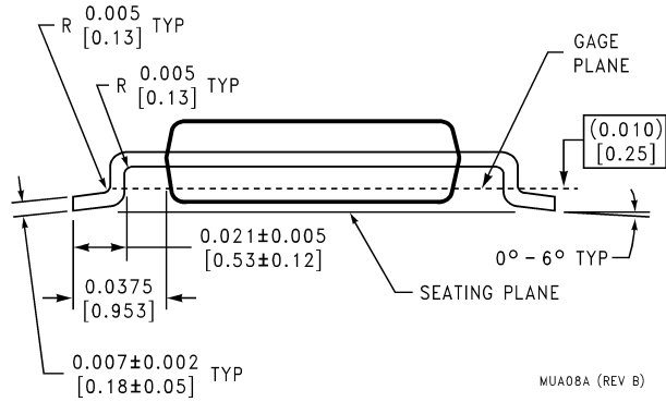
Mini SO-8 Package NS Package Number MUA08A
