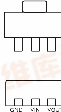
C. SOT-89
