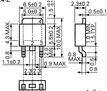
2SJ324-Z
