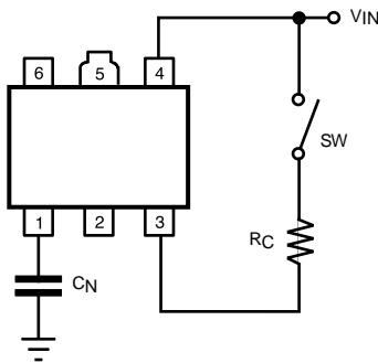
SOT-89
