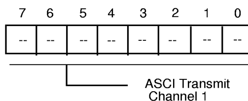
Figure 37. ASCI Register
