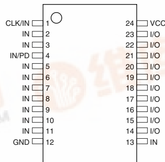
TSSOP
