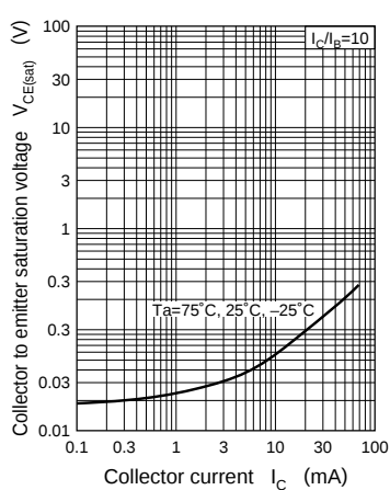
V_{CE(sat)} - I_C
