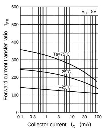
h_{FE} - I_C
