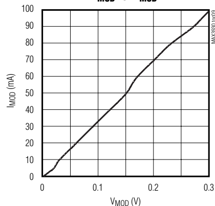
I_{MOD} vs. V_{MOD}
