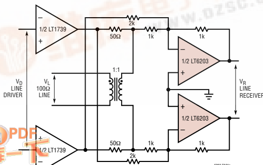
低噪声四线至双线本机回波抵消差分接收机
