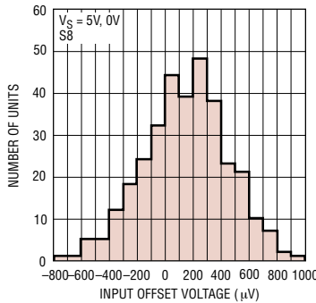
V_{OS} 分布, V_{CM} = V^+
