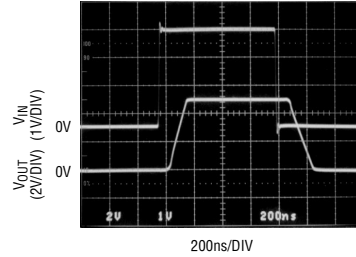
输出过载恢复
