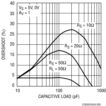
串联输出电阻与容性负载的关系曲线
