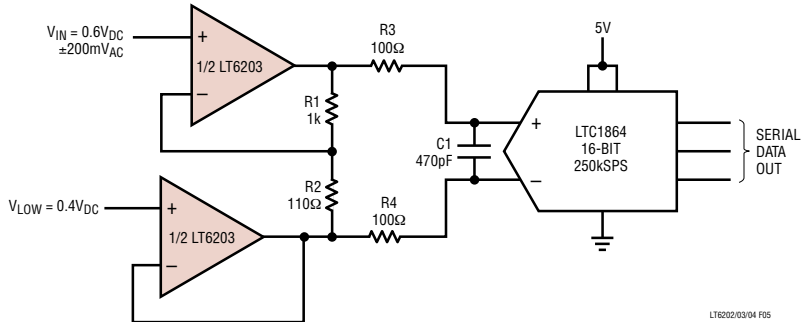
图 5：单电源 16 位 ADC 驱动器
