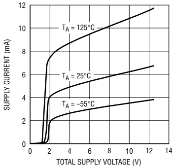
供电电流与电源电压的关系 (两个放大器)
