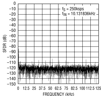
图 6：显示 100dB SFDR 的 FFT
