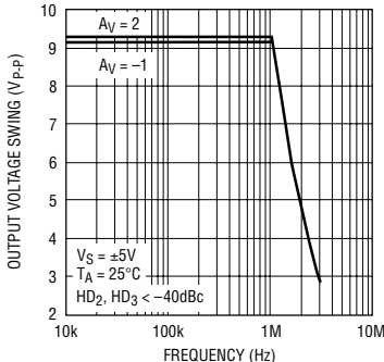
最大失真输出信号与频率的关系曲线
