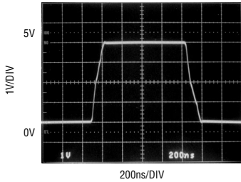
5V 大信号响应
