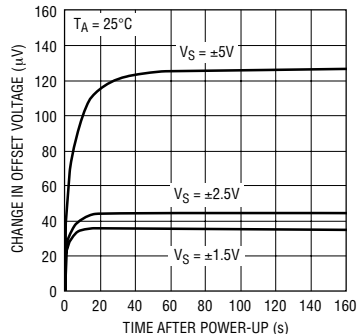
温升漂移与时间的关系曲线 (LT6203S8)
