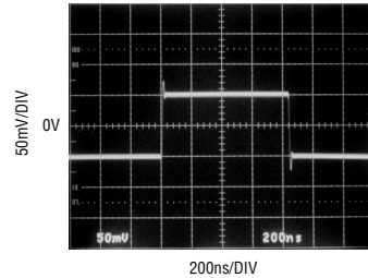
5V 小信号响应
