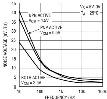
输入噪声电压与频率的关系
