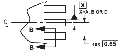
VIEW Y
